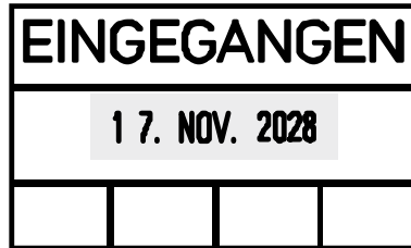
2910/P04/C6 54 x 30 mm | max. Textplattengröße 4 mm | Schrifthöhe Datum
