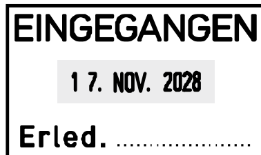
2910/P04/C9 54 x 30 mm | max. Textplattengröße 4 mm | Schrifthöhe Datum
